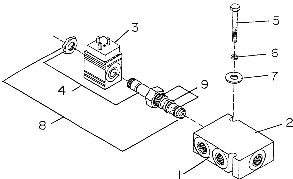
ASSEMBLY ITEMS 2,3,4
